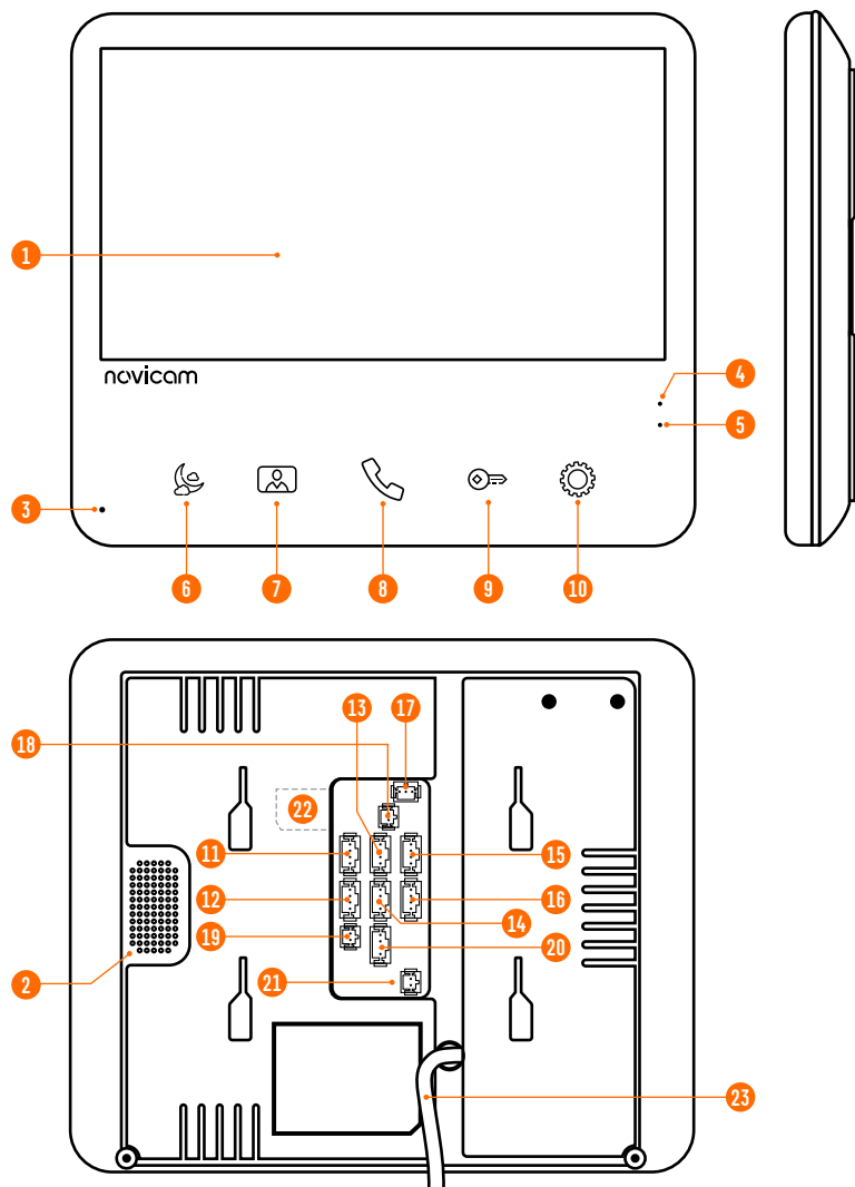
Рис. 2 Видеодомофон UNIT 7 FHD
