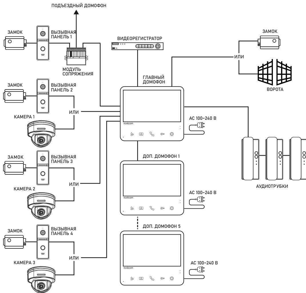
Рис. 11 Структурная схема системы на базе видеодомофонов UNIT 7 FHD
