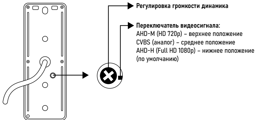
Рис. 8 Регулировка громкости динамика и выбор типа видеосигнала
