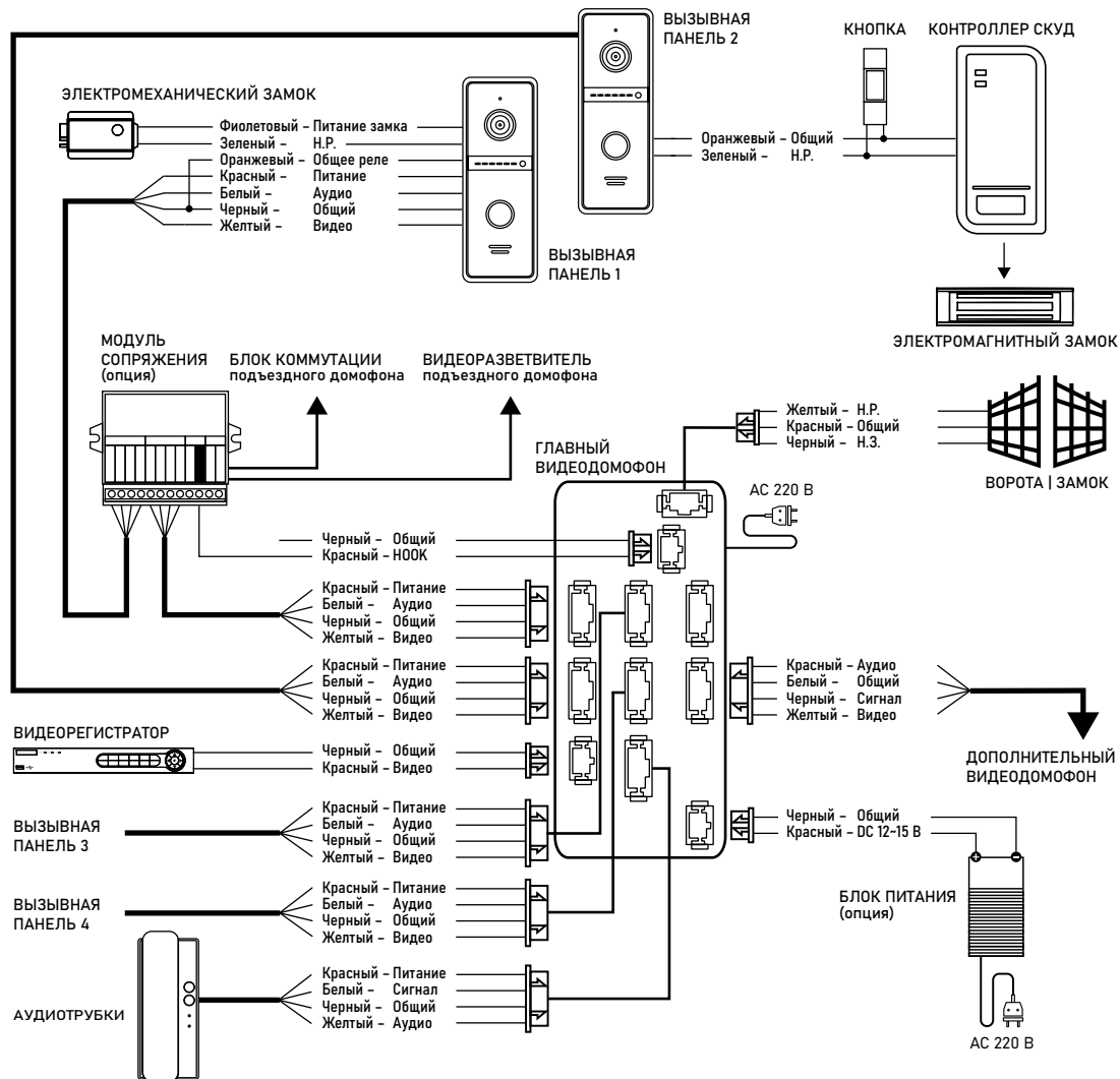
Рис. 12 Общая схема подключения видеодомофонов серии UNIT FHD
