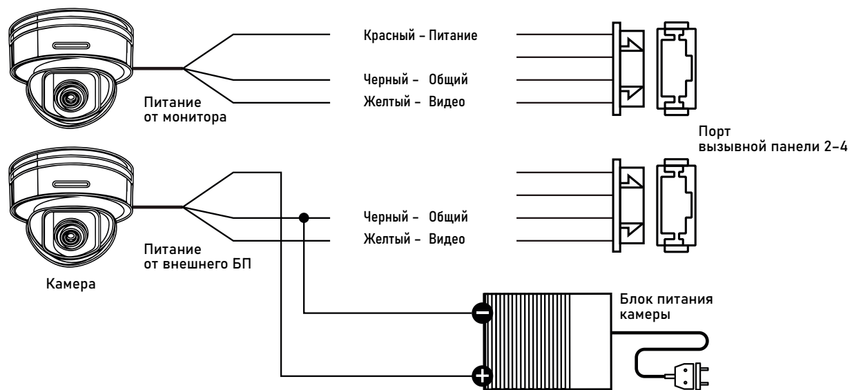
Рис. 14 Схема подключения видеокamеры к домофону UNIT FHD
