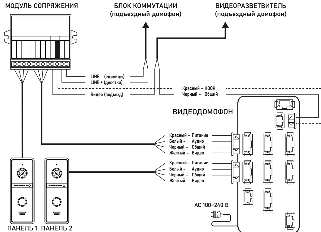
Рис. 13. Схема подключения видеодомофонов серии UNIT FHD к подъездному домофону через модуль сопряжения
