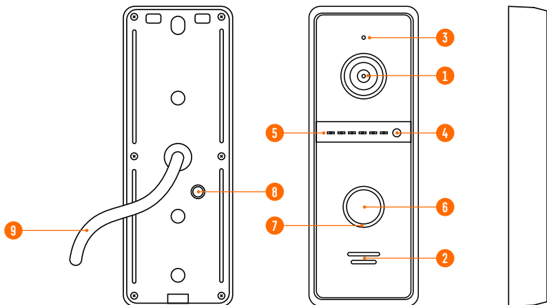
Рис. 3 Вызывная панель, входящая в комплект UNIT 7 FHD KIT
