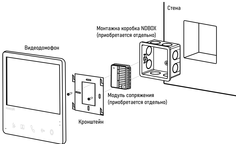
Рис. 5 Монтаж видеодомофона UNIT 7 FHD
