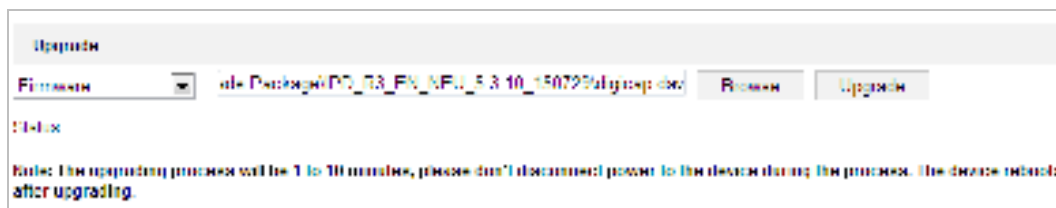
Рисунок 6-47 Удаленное обновление системы
