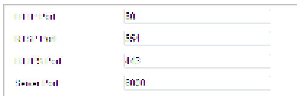
Рисунок 6-7 Настройка портов
