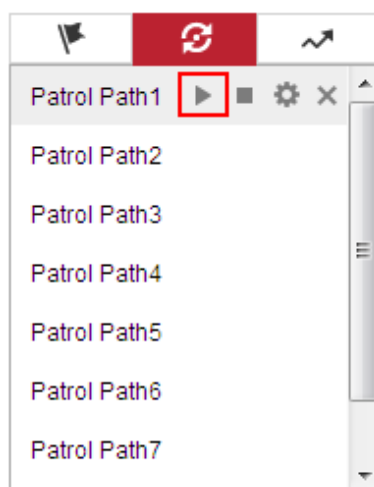
Рисунок 4-10 Вызов патруля
