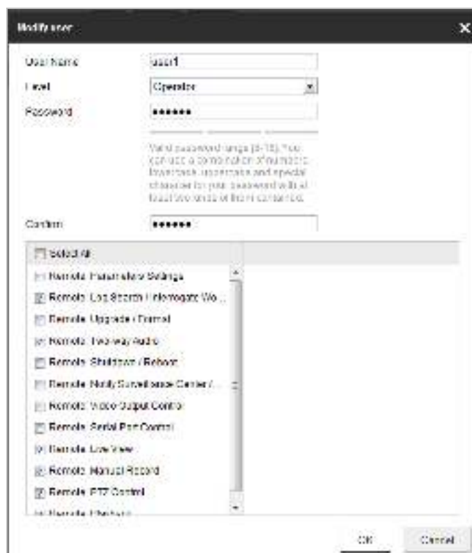
Рисунок 6-55 Редактирование пользователя
