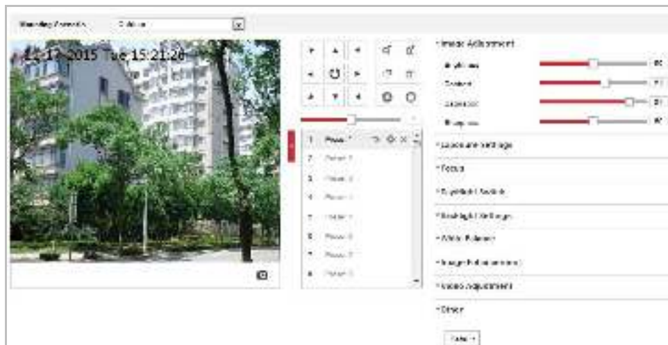
Рисунок 6-25 Настройки отображения
