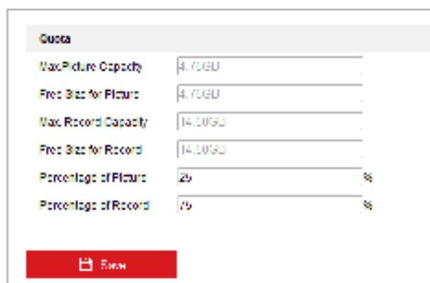
Рисунок 5-10 Настройка квоты
