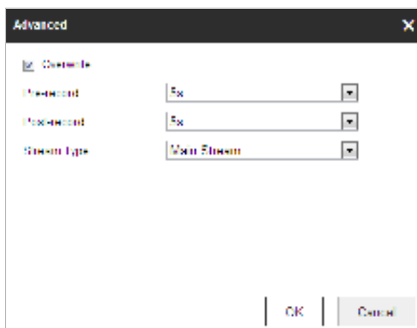
Рисунок 5-2 Параметры записи
