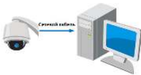
Рисунок 2-1 Подключение напрямую
