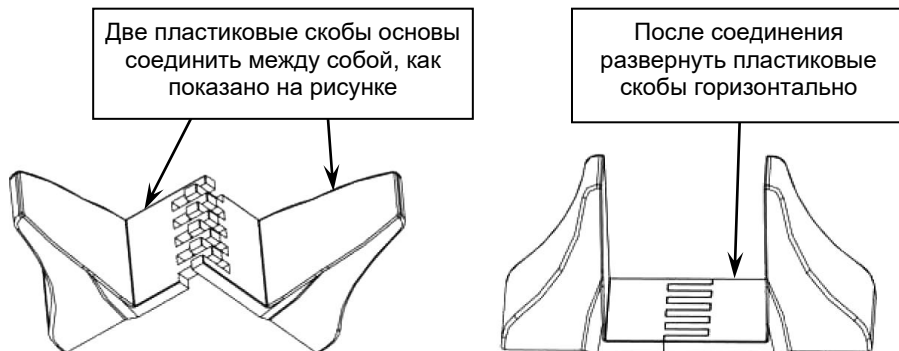
Рисунок 3 – Сборка пластиковых основ для вертикальной установки изделия
