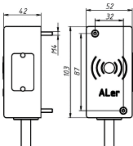
Рисунок 1 - Габаритно-установочные размеры счетывателя AL-RD-05 (вариант К)
